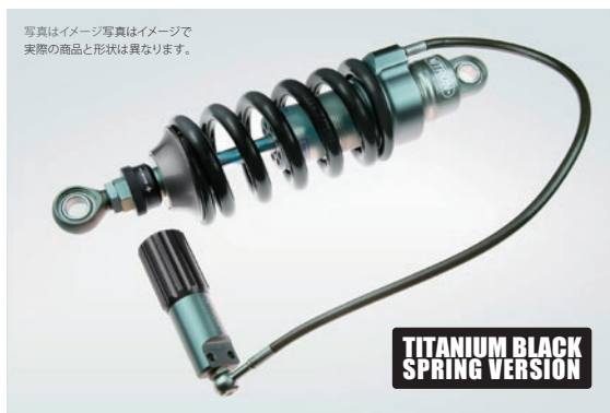
R1 Series 標準価格 ¥137,500 (税込) NTBKY78S-TB 1way ダンピングアジャスター搭載 / 内蔵リザーバタンクモデル 油圧式プリロードアジャスター標準装備モデル
